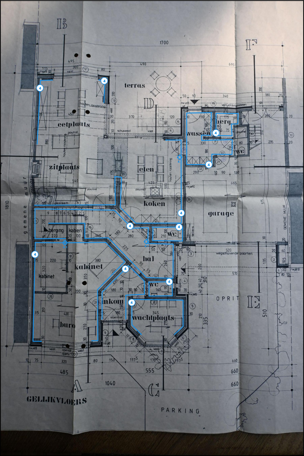
Legende van plan 1.1: Grondplan
